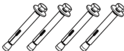
Монтаж из нержавеющей стали винты M8×80 x4
